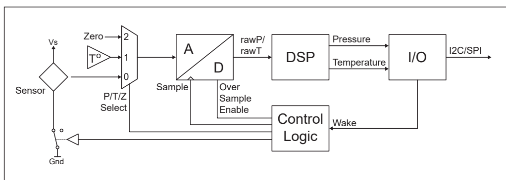
図 1 - DLVの本質モデル
